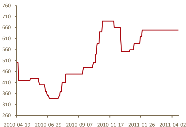
图表 29 国内硫酸（华东 98%）走势（元/吨）
