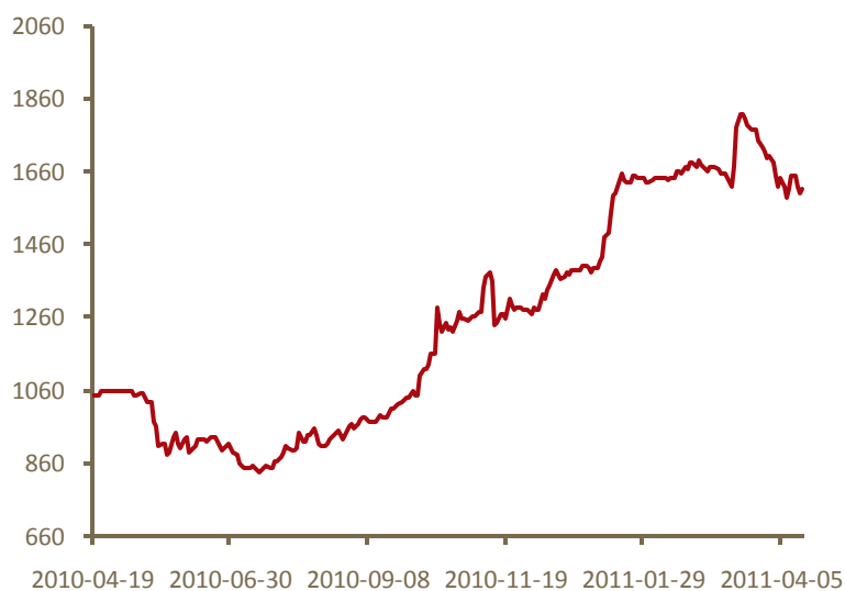
图表 28 PX（进口到岸价）价格走势（美元/吨）
