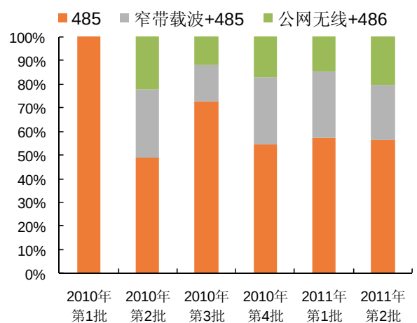
图表6 三相电表(1S级)历次招标通信方式比例
