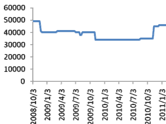
图 35: 长三角顺丁橡胶价格走势
