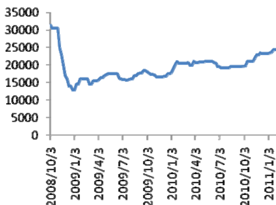
图 33: 长三角丁腈橡胶价格走势
