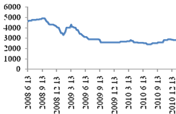
图 38: 长三角市场钾肥价格走势图
