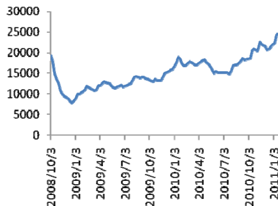
图 32: 长三角丁苯橡胶价格走势走势图
