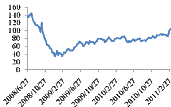
图 6：本周长三角市场纯苯价格走势
