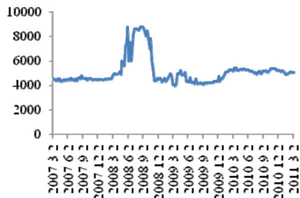
图 22：长三角市场磷酸价格走势
