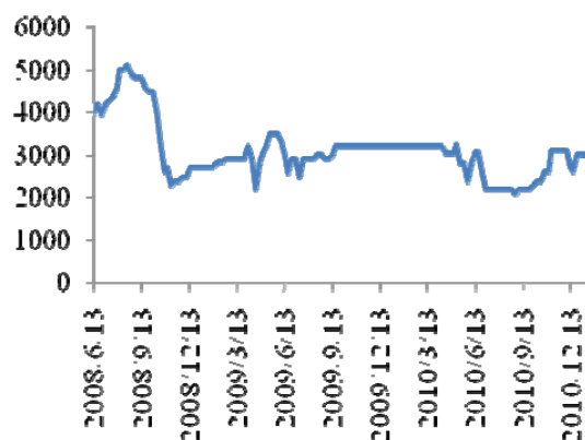
图 13：长三角市场硝酸价格走势
