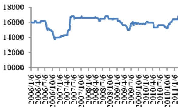
图 29: 长三角聚甲醛价格走势走势图
