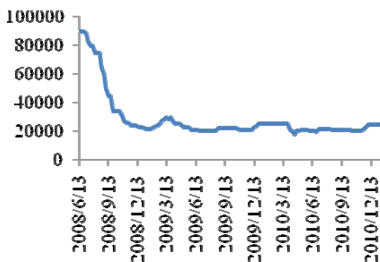
图 36: 长三角市场草甘膦价格走势
