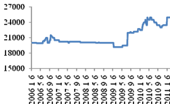
图 30: 长三角PBT价格走势走势图
