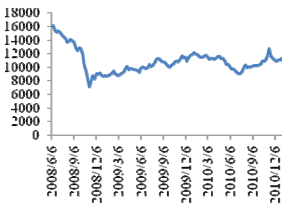
图 25：本周长三角市场PS价格走势
