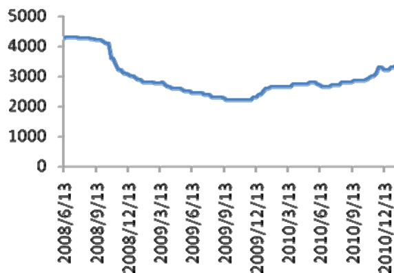
图 39: 长三角市场磷肥价格走势图
