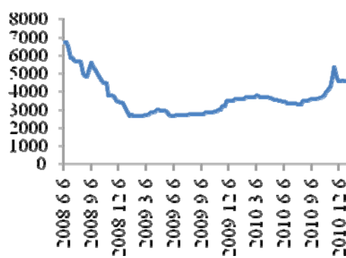
图 19: 长三角市场二甲醚价格走势
