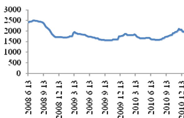
图 37: 长三角市场尿素价格走势
