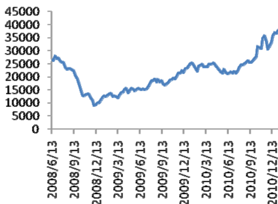
图 31: 天然橡胶上海期货价格走势走势图
