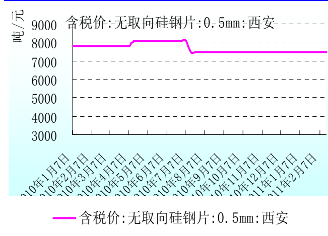
图 15 硅钢（50ww800）周价格走势图
