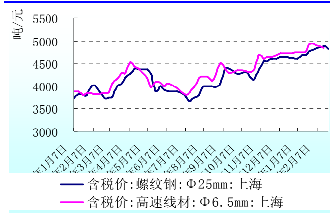
图 11 上海地区建筑用钢价格走势图
