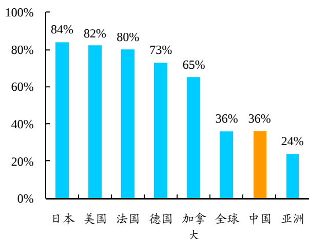
图 12: 2007 年部分国家水电开发程度比较
