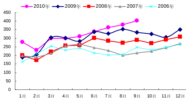
图 13：中国精炼铅产量（2006-2010）KT
