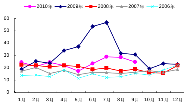
图 23：中国镍表观消费（2006-2010）KT
