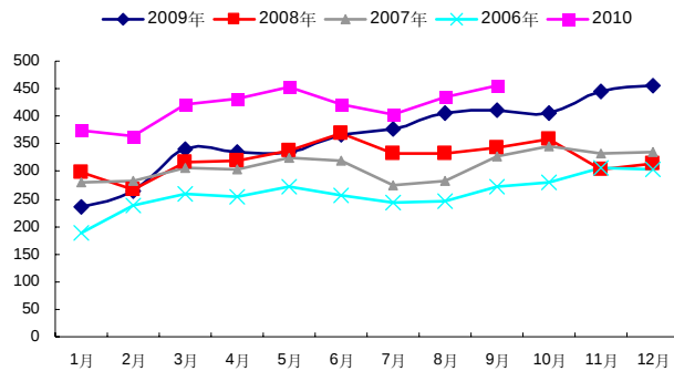
图 17：中国精炼锌产量（2006-2010）KT
