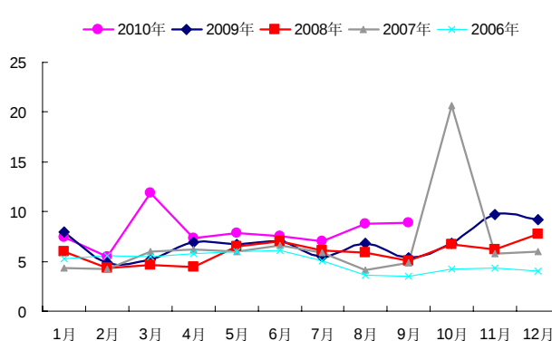
图 22: 中国锡精矿供应 (2006-2010) KT
