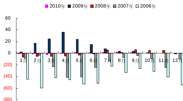
图 14：中国精炼铅净进口（2006-2010）KT
