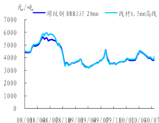
图 5: 螺纹钢均价上涨 3.18%; 高线均价上涨 3.27%
