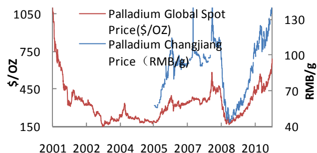
图 22. 国际现货与长江钯价格
