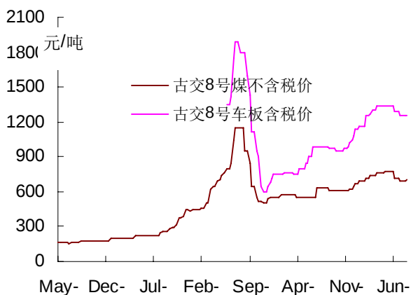
图 21: 古交 8 号焦煤价格走势
