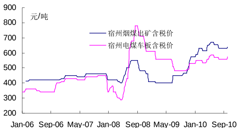
图 5：宿州烟煤、电煤价格走势
