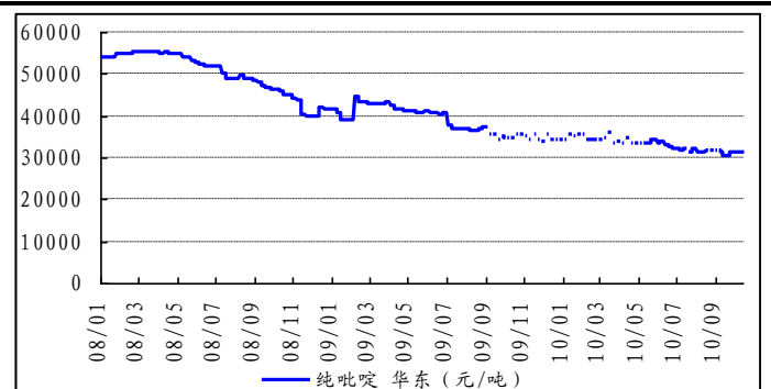
图2: 国内吡啶价格
