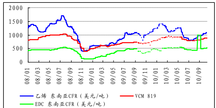
图2: 乙烯、EDC及VCM东南亚到岸价
