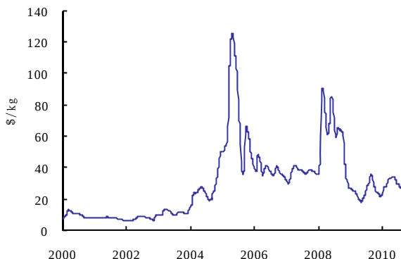
图 38. 欧洲钒 70-80%价格
