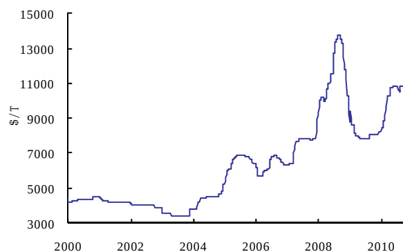
图 34. 国际铬 99%价格
