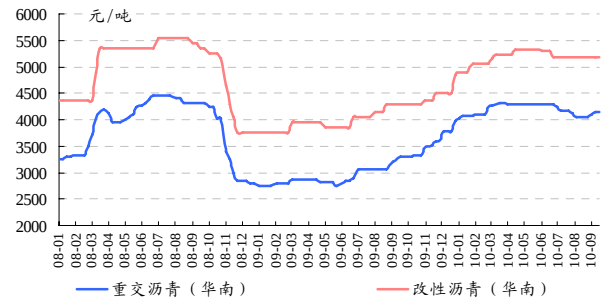
图 54 沥青价格
