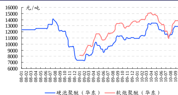
图 37 聚醚价格
