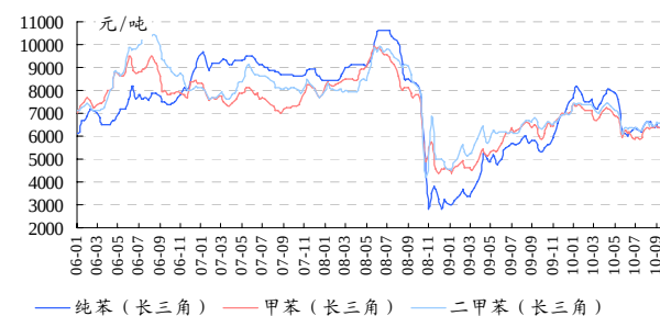
图10 芳烃价格
