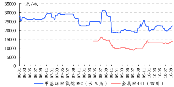
图 52 有机硅价格
