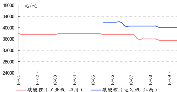
图 55 碳酸锂价格
