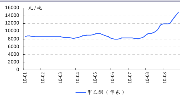
图 41 甲乙酮价格
