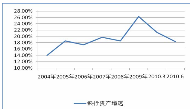
图3 中国银行业资产增速
