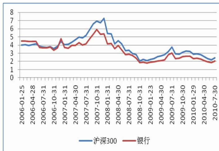
图2 银行股及沪深300指数P/B
