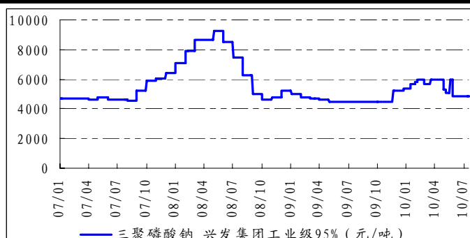
图6: 国内三聚磷酸钠价格
