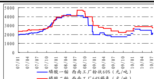
图3: 国内磷酸一铵、二铵价格
