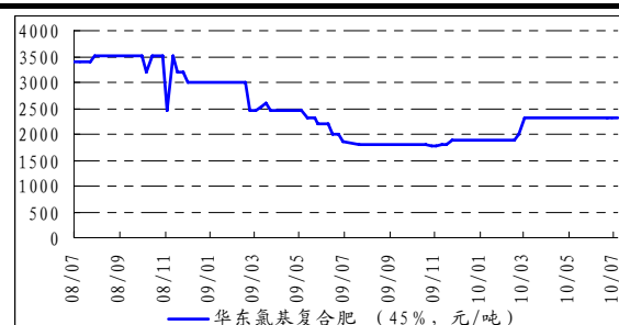
图4: 国内氯基复合肥价格
