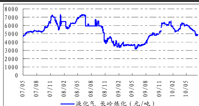
图6：国内液化石油气
