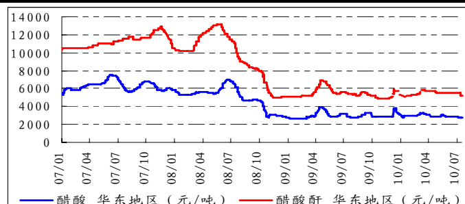
图4：华东地区醋酸、醋酐价格
