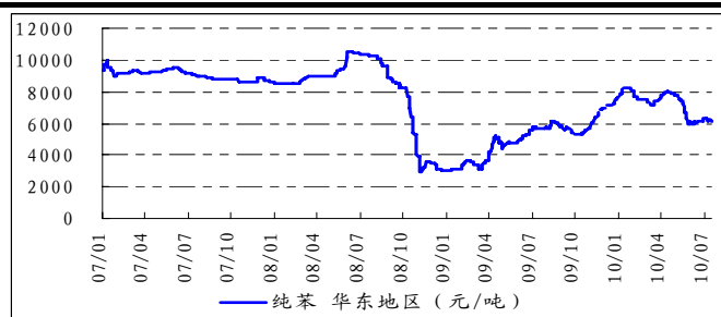
图1: 国内苯价格走势
