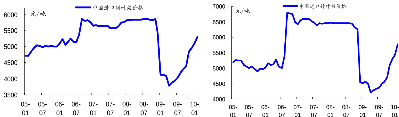
图表 4: 进口纸浆价格走势
