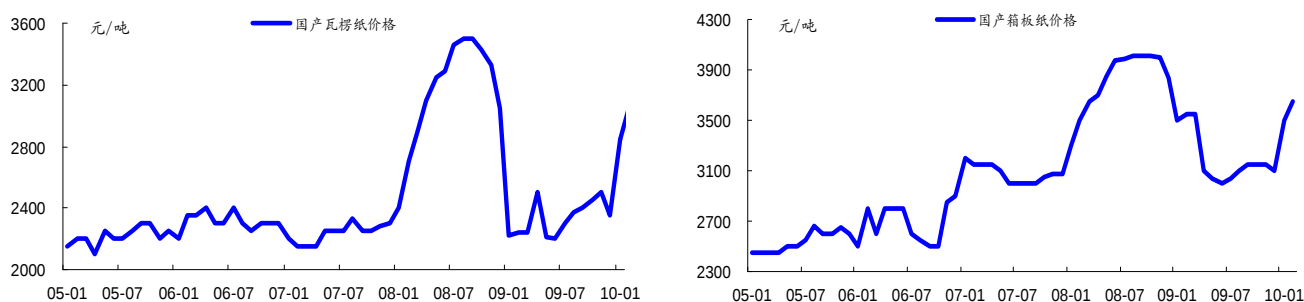
图表 2：国产瓦楞纸及箱板纸价格走势（中国纸网最新数据还没有公布）
