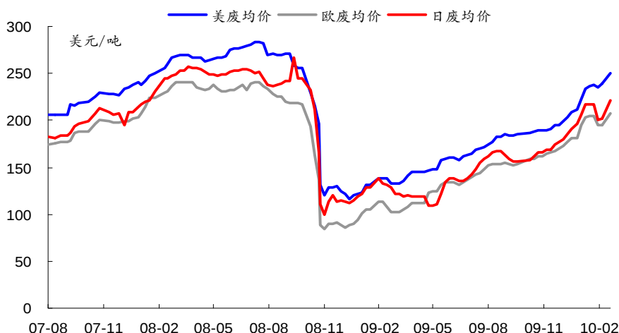
图表 3：进口废纸价格走势
