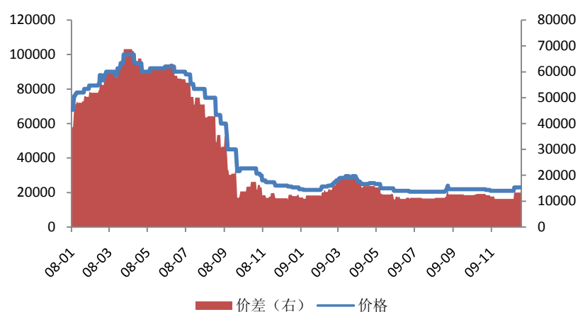
图 22: 草甘膦(二乙醇胺)价格与价差
