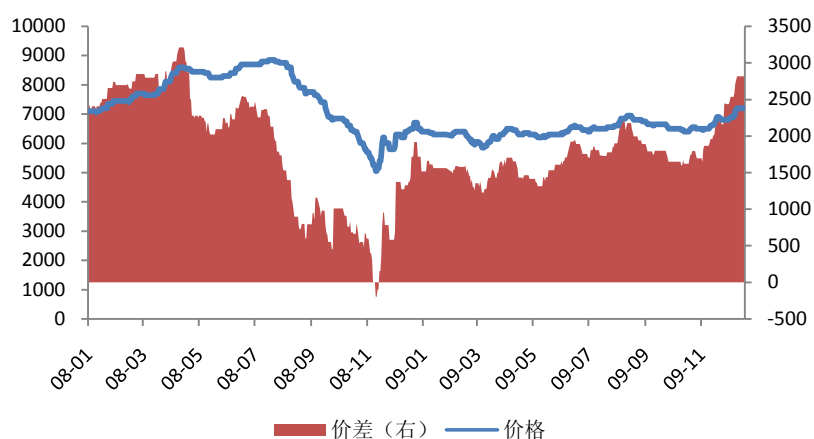
图 3: PVC(电石法)价格与价差
