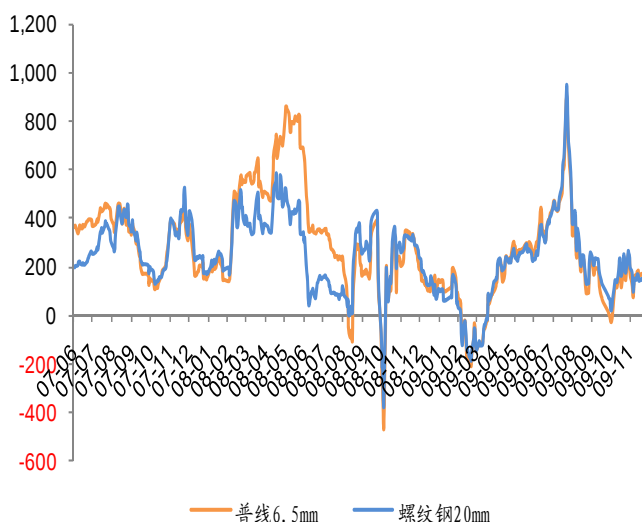
图22：普线、螺纹钢毛利走势（单位：元/吨）
