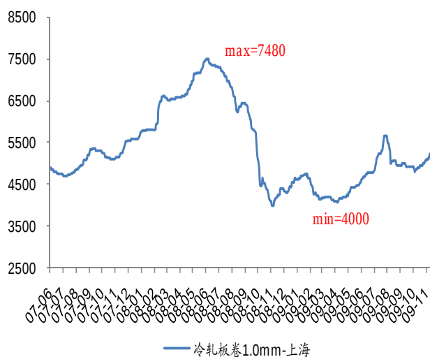
图10: 中板价格走势 (单位: 元/吨)
