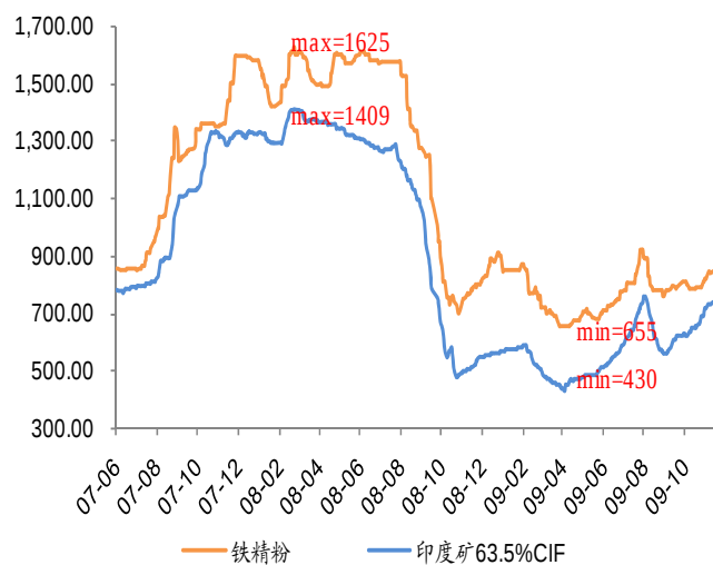
图2: 国内铁精粉和印度矿价格走势 (单位: 元/吨)
