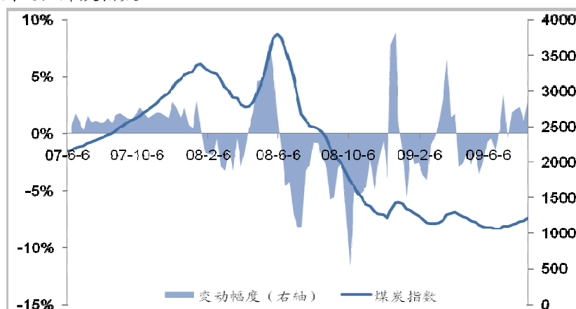
图 3: 煤炭指数
