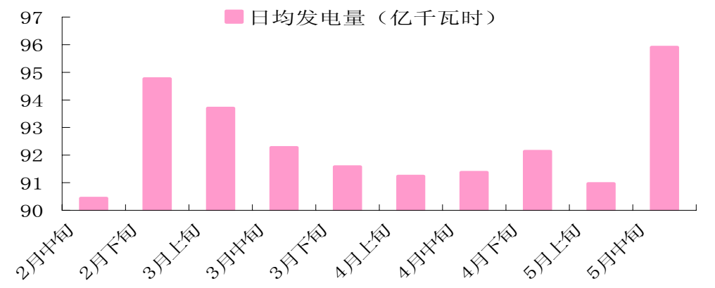
图6 2009年春节后日均发电量趋势
