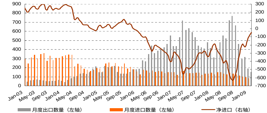
图表2. 08年四季度开始我国钢材出口量持续下滑 单位：万吨
