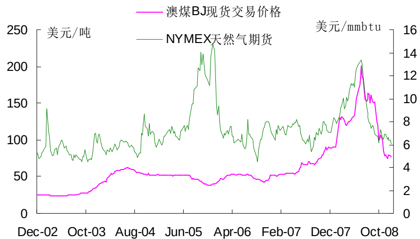
图 45: NYMEX 天然气期货价格
