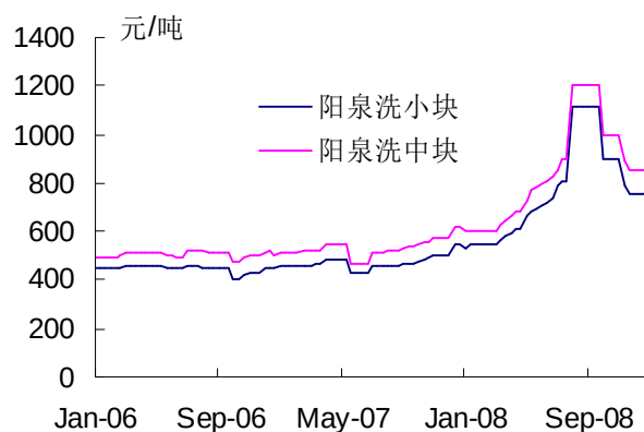
图 27：阳泉块煤价格
