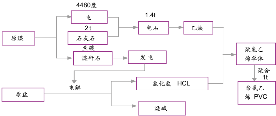
图9：煤头PVC产业链图（物料消耗以行业平均计算）
