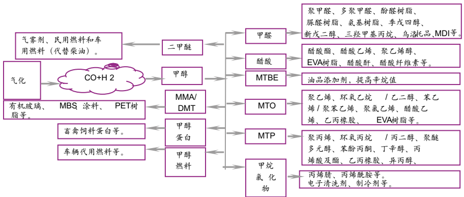
图13：甲醇衍生品产业链
