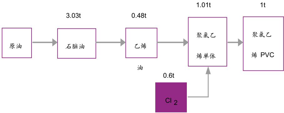
图10：油头PVC产业链（物料消耗以行业平均计算）
