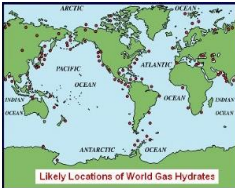
图 6：世界天然气水合物资源情况
