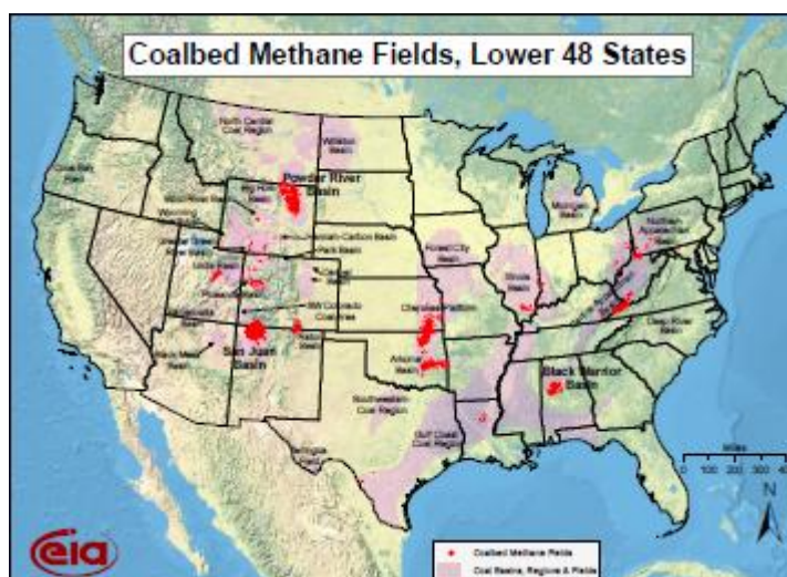
图 5：美国煤层气资源情况（2009）
