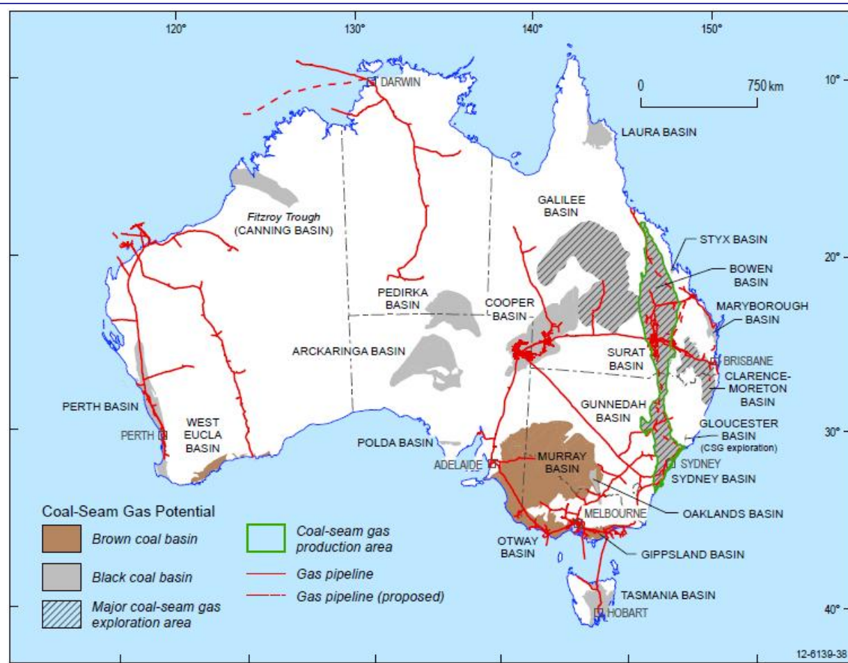
图 4：澳大利亚煤层气资源情况 (2012)
