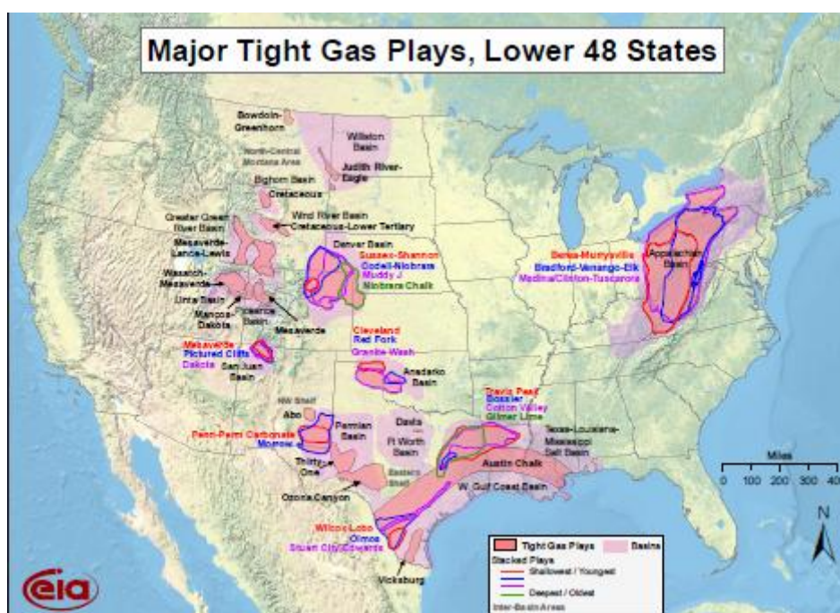
图 1: 美国致密气资源情况 (2010)
