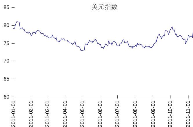
图 6：美元指数小幅下跌，但仍处于高位，由于意大利债务危机初严重，对其避险需求依然强劲。
