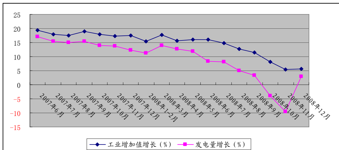
图2 08年12月发电量的触底回升预示中国经济出现企稳反弹迹象
