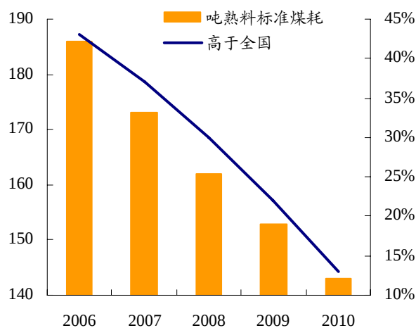
图 10: 新疆吨熟料标准煤耗及高于全国幅度
