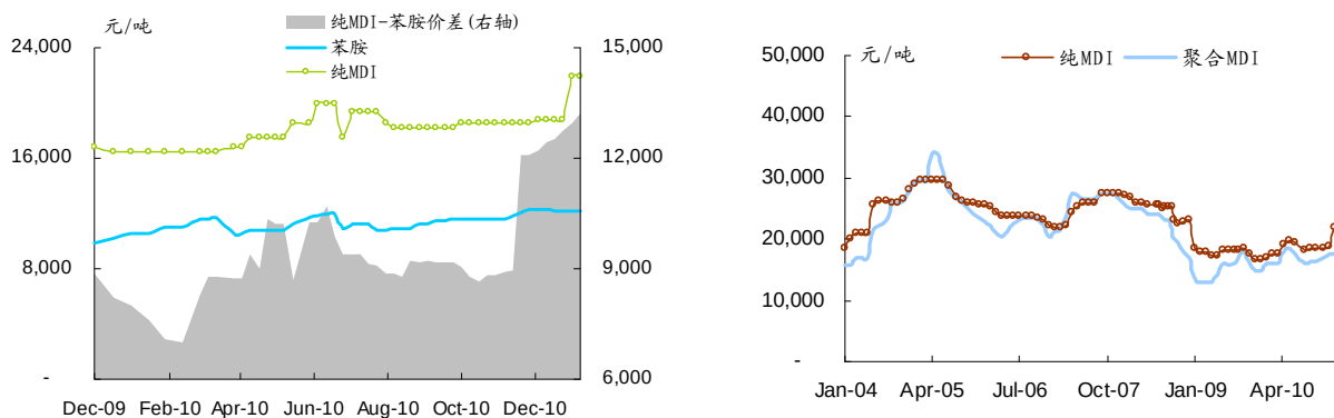
图表 1: 纯 MDI 与苯胺价差走势 (左); MDI 价格走势 (右)
