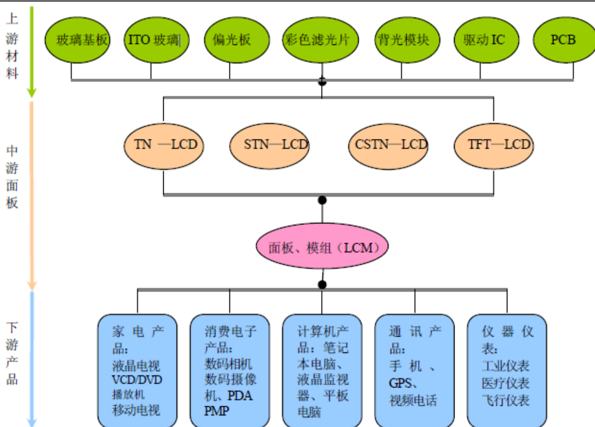
图 4: LCD 产业链
