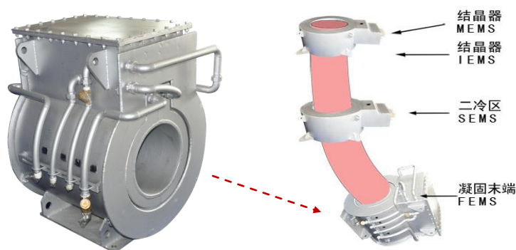
图表 10 圆坯结晶区 EMS 实物图
