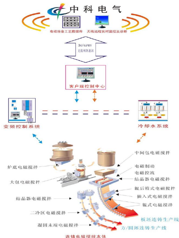
图表 21 公司连铸电磁冶金整体解决方案示意图
