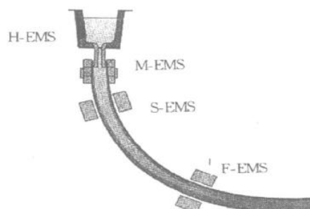
图表 9 连铸机电磁搅拌的位置
