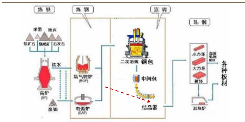
图表 6 连铸在钢铁工艺流程中的位置
