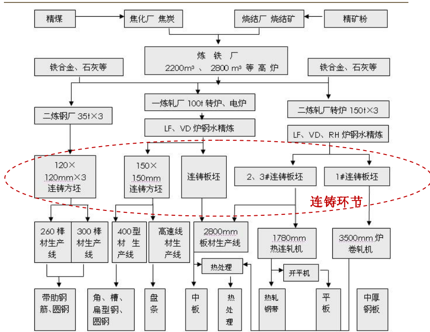
图表 7 国内某大型钢铁厂生产线结构图
