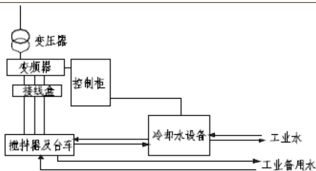
图表 18 电磁搅拌系统示意图
