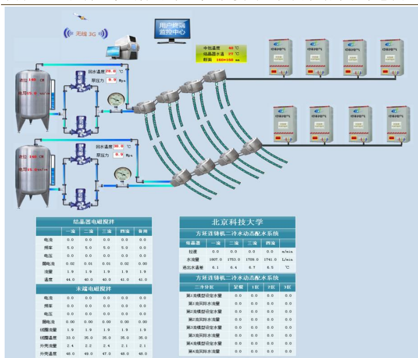
图表 22 公司在线运行产品无线远程实时监控及诊断系统示意图
