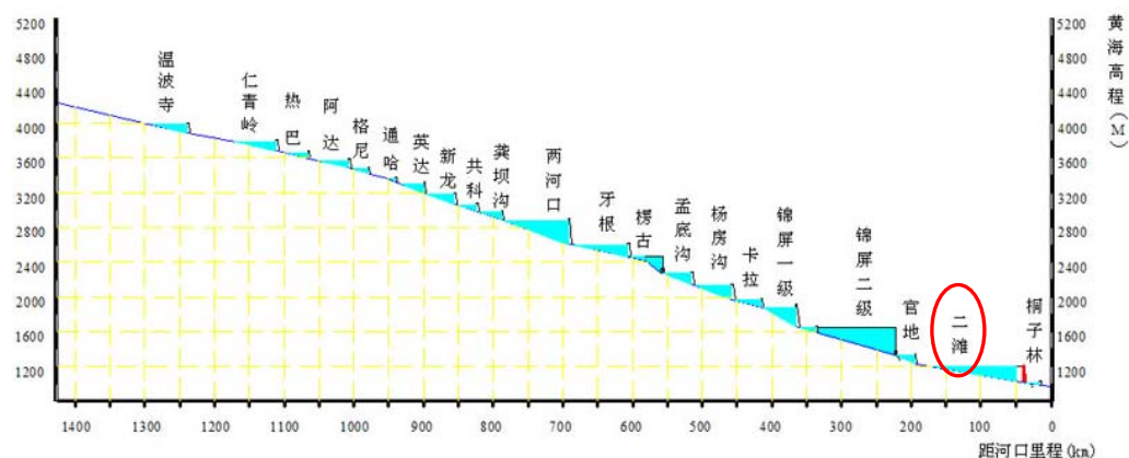
图 4 二滩梯级电站建设剖面图
