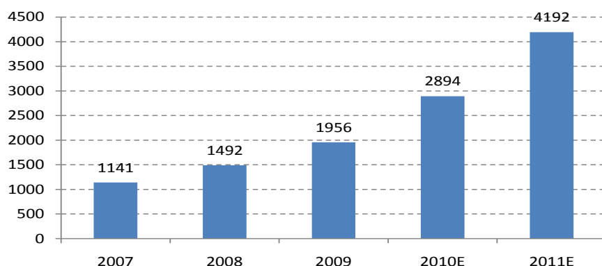
图5. 全球海上风电累计装机容量 (MW)
