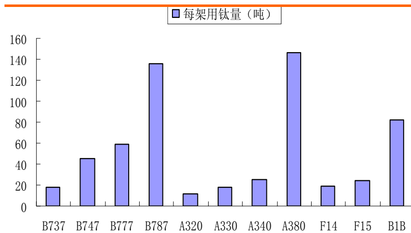
图 7 飞机的钛材应用量现状
