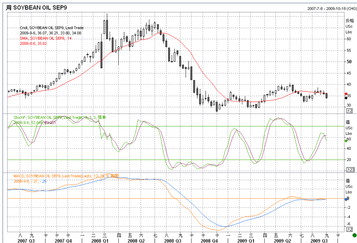
9 月豆油周线图
