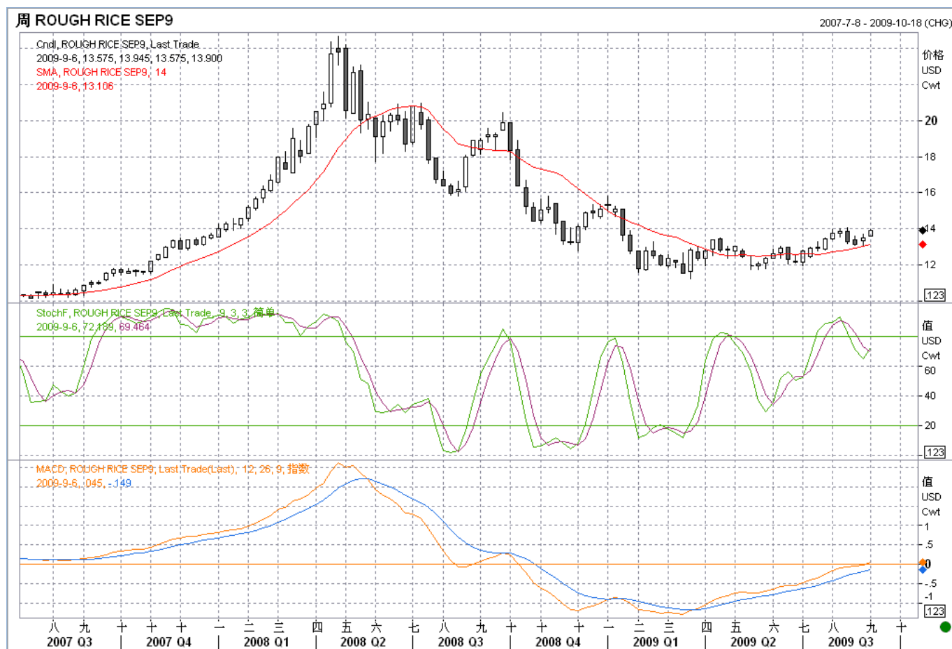
9 月稻米周线图
