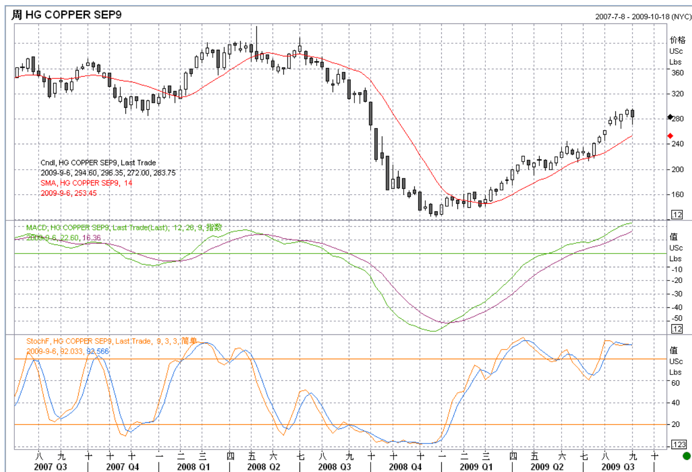
9 月期铜周线图
