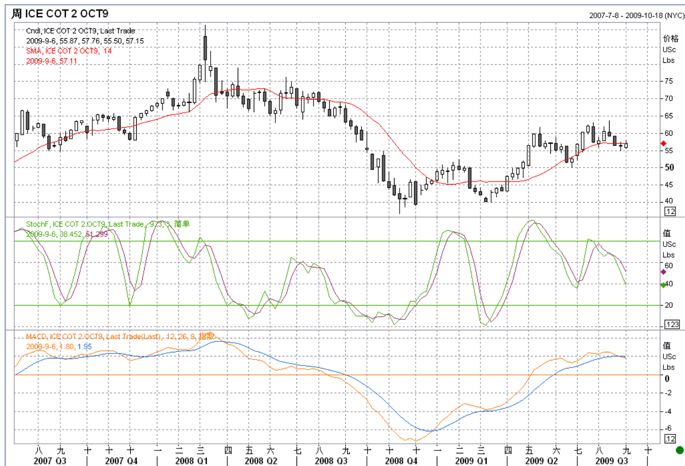
10 月期棉周线图
